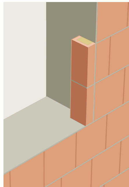
Laibung und Brüstung mit Mörtel abgleichen.
