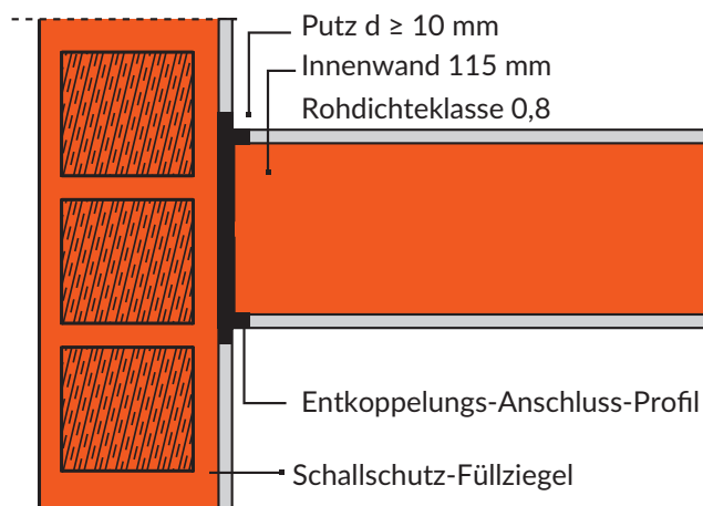
Bild 22: ZIS - Ziegel-Innenwand-System
