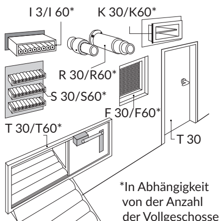
Bild 19: Verschlüsse in F 90 Wänden
