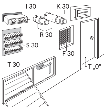
Bild 18: Verschlüsse in F 30 Wänden
