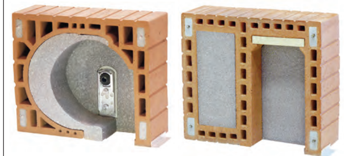
Bild 15: Ziegel-Rollladenkasten (Beispiele)
