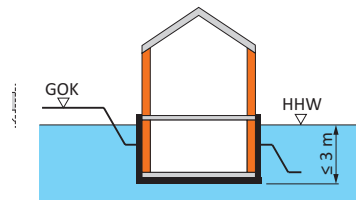
W2.1-E | Hohe Einwirkung von drückendem Wasser
