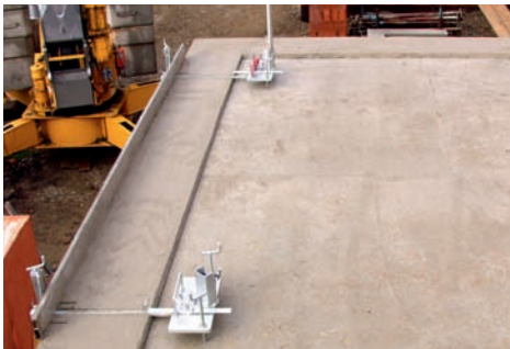
1. Anlegen des Mörtelbettes mit einer Justiereinrichtung
