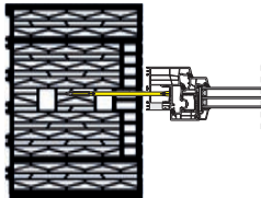
Bild oben und Mitte: Hygrothermisch optimaler, mittlerer Fensteranschluß bei ganzem Ziegel mit keramisch verstärktem Kern in der ersten Schicht.
