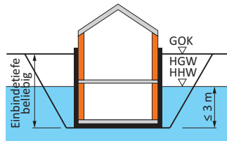
W2.1-E | Grundwassereinwirkung \leq 3 m
