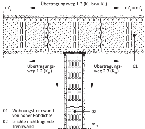
Darstellung der Schallübertragungswege eines sogenannten T-Stosses am Beispiel einer mit ZIS bauakustisch entkoppelt angeschlossenen nichttragenden Trennwand an eine Wohnungstrennwand aus mit Beton vergessenen Planfüllziegeln
