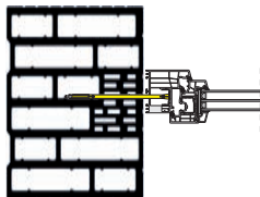
Bild unten: Fensteranschluß mit Halbstein in der zweiten Schicht und mit optionaler Anschlagsschale außenseitig.
