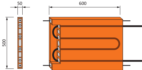
Ziegelheizelement: Langlochziegel mit integriertem Heizstrang
