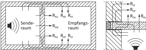
Schallübertragung über das trennende Bauteil ( R_{Dd,w} ) und die flankierenden Bauteile ( R_{Fp} , R_{Fd} , R_{Df} ) horizontal und vertikal
