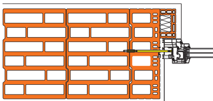
Bild unten: Fensteranschluß mit Halbstein in der zweiten Schicht und mit optionaler Anschlagsschale außenseitig.
