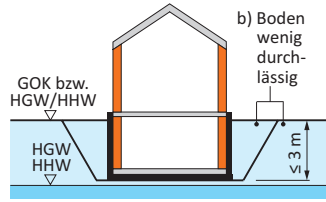
W2.1-E | Stauwasser \leq 3 m, ohne Dränung
