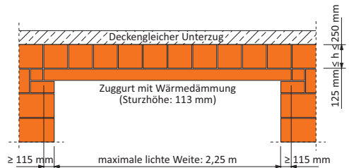
Geometrische Randbedingungen für Flachstürze mit 113 mm hohen Zuggurten mit Wärmedämmung und einlagiger Übermauerung
